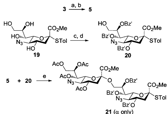
Scheme 3. a) NBS, acetone/H 2 O, RT, 1 h, 91 %. b) NEtPr 2 , CIP(OEt) 2 , CH 3 CN, RT, 30 min, 65 %. c) t BuMe 2 SiCl, py, DMAP, CH 2 Cl 2 , RT, 1 h, then Bz'Cl, 0 °C to RT, 1 h, 88 %. d) HF/py, AcOH, THF, 1 h, 89 %. e) TMSOTf, 3 Å MS, CH 3 CN, –40 °C, 30 min, 51 %.
